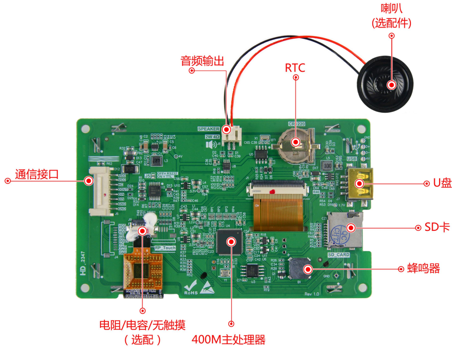
图 1-4 硬件配置图
