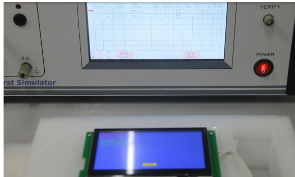
图 4-3 EFT 测试图
