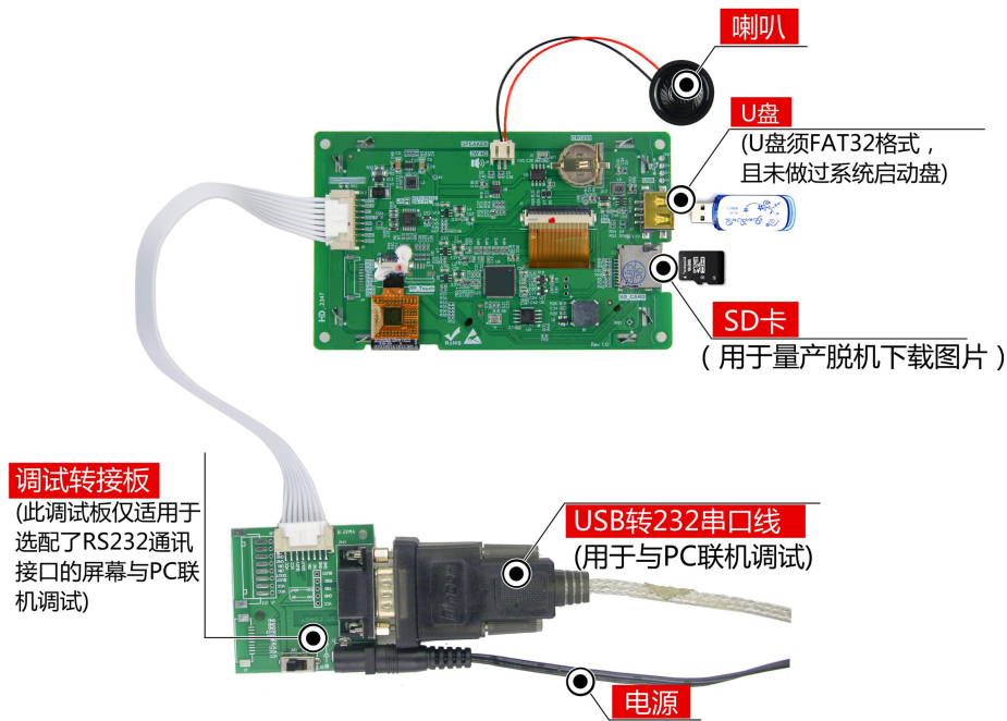
图 1-5 RS232 调试图
